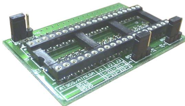
Gambar 5. Soket Konverter untuk AVR ® 40-pin
