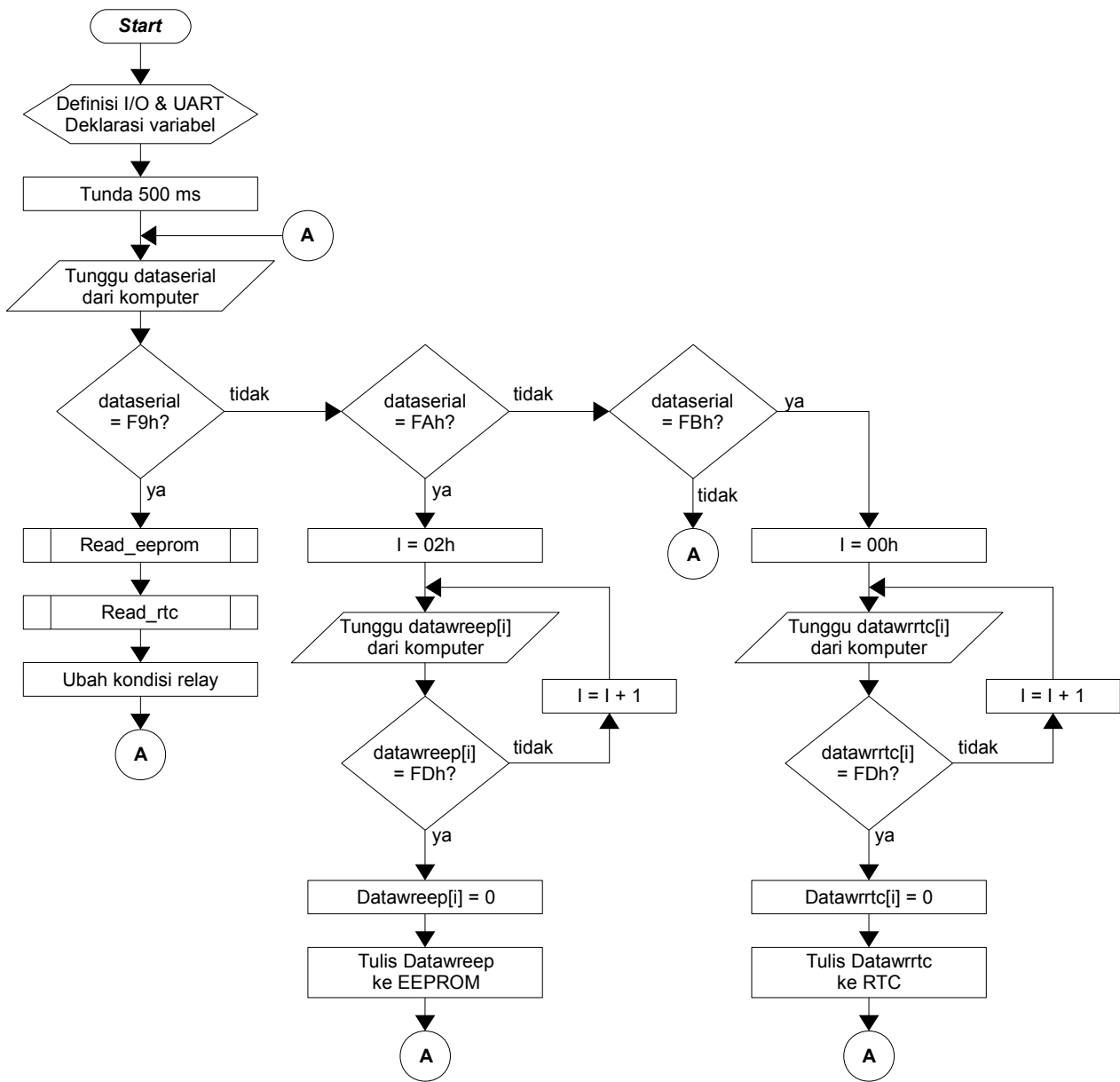
Gambar 2 Flowchart Program Terakhir.BAS
