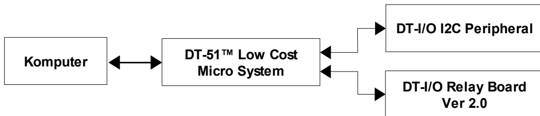
Gambar 1 Blok Diagram AN146
